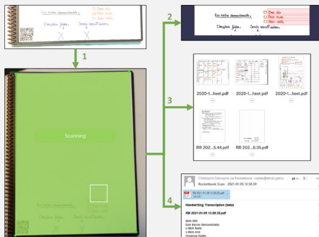
Figuur 1: Men vinkt de bestemming van notities aan (hier Dropbox en email). Na het scannen (1), zal de app lijsten herkennen (2), het bestand in een Dropbox folder opslaan (2), en een email met bijlage verzenden (3). De email bevat ook de tekst van de scan gebruikmakende van OCR.
